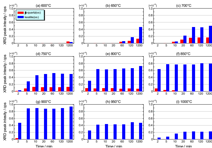
LAS-Ca 結晶化ガラスからの結晶析出挙動
