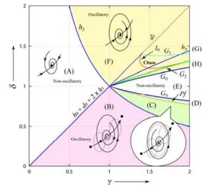
分岐図
